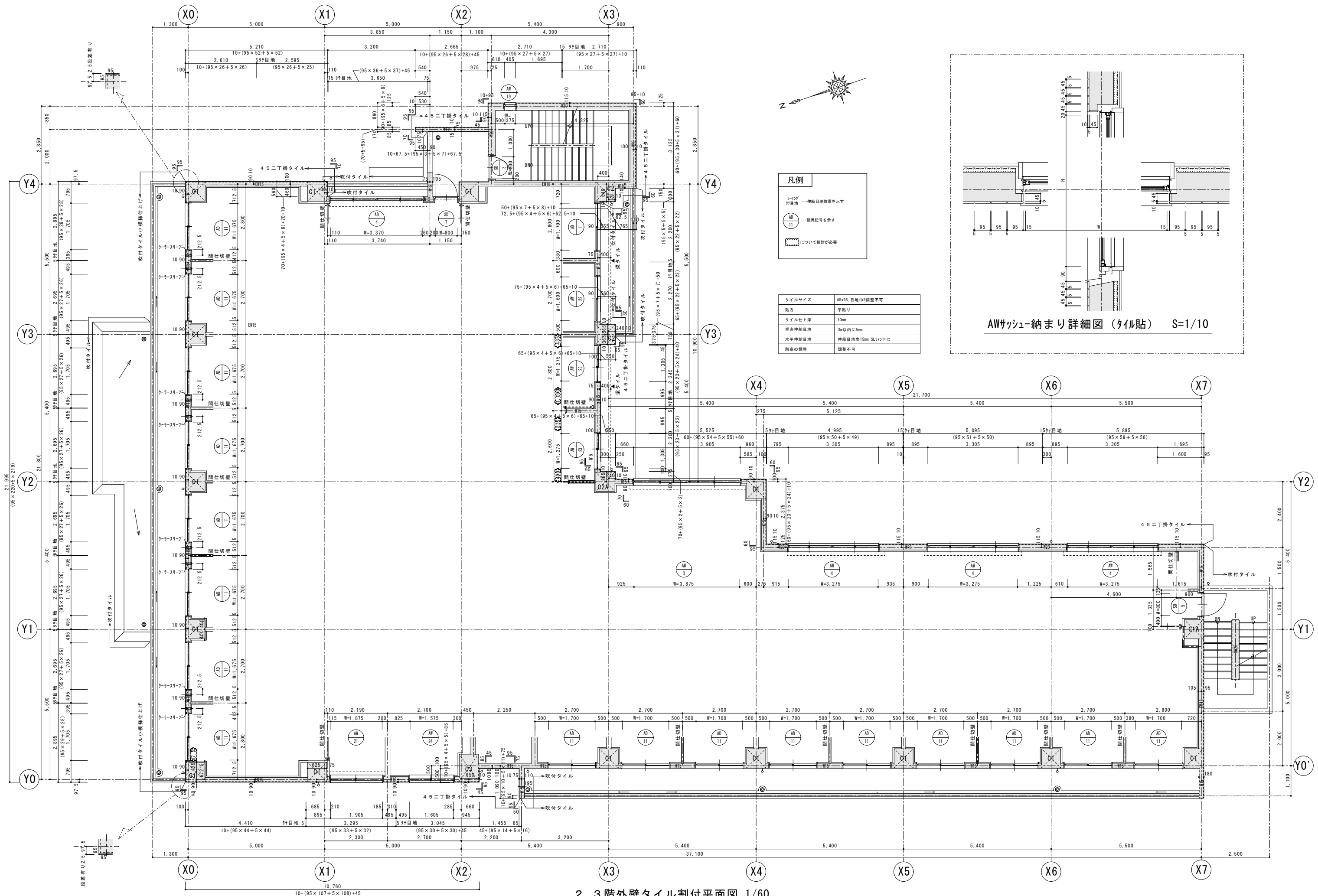
2, 3階外壁タイル割付平面図 1/60
